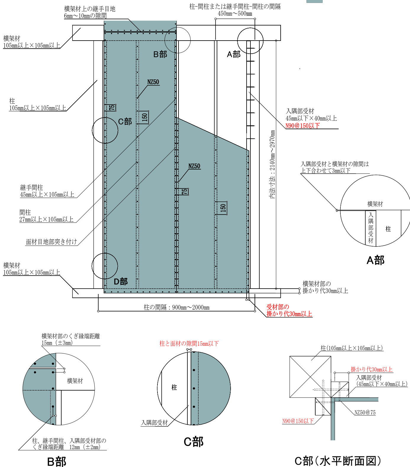
図 11 入隅仕様 (FRM-0734 : 2.7 倍) 施工概略図 (2P の場合)
