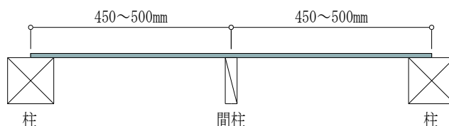
図 24 1P 耐力壁 納まり図
