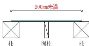
図27 狭小幅の壁 納まり図
